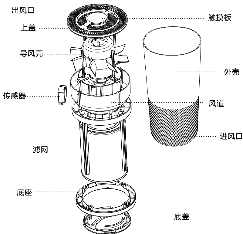
产品爆炸图
